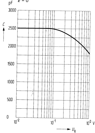
Sperschicht-Kapazität C = f(U_R) E = 0
