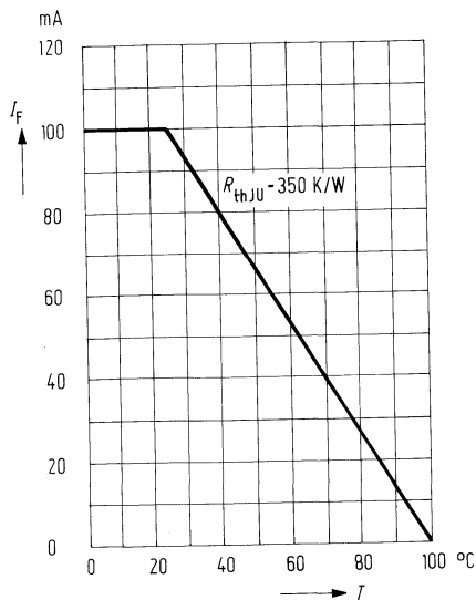
Maximal zul. Durchlaßstrom
