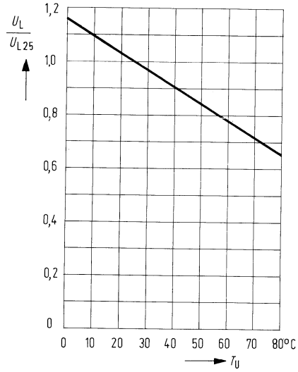
Leerlaufspannung U_L = f(T_U)
