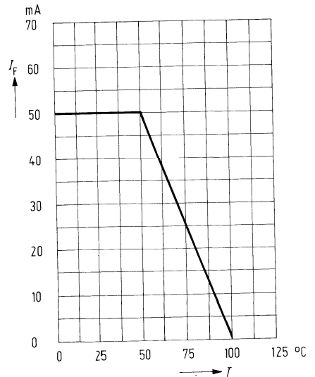
Maximal zulässiger Durchlaßstrom I_F = f(T)
