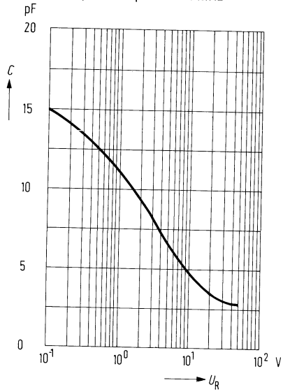
Sperschichtkapazität C = f(U_R) E = 0 ; Meßfrequenz f = 1\text{ MHz}
