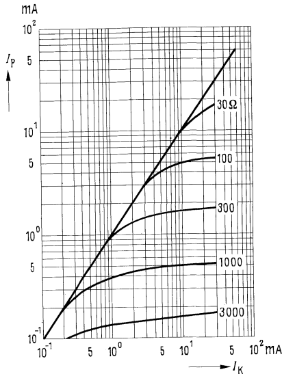
Fotostrom in Abhängigkeit vom Kurzschlußstrom I_p = f(I_k) R_L = \text{Parameter}
