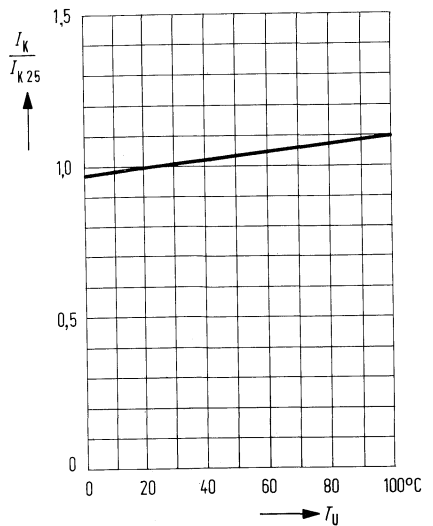
Temperaturabhängigkeit von I_K
