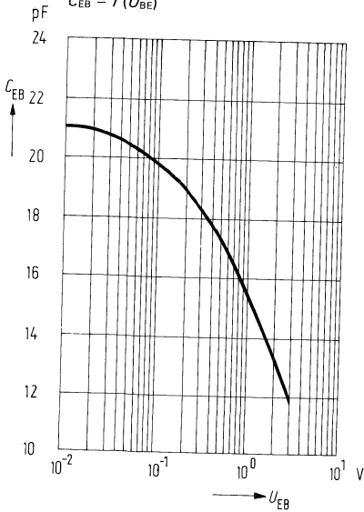
Emitter-Basis-Kapazität C_{EB} = f(U_{BE})
