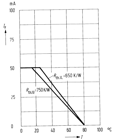
Maximal zul. Durchlaßstrom I_F = f(T)
