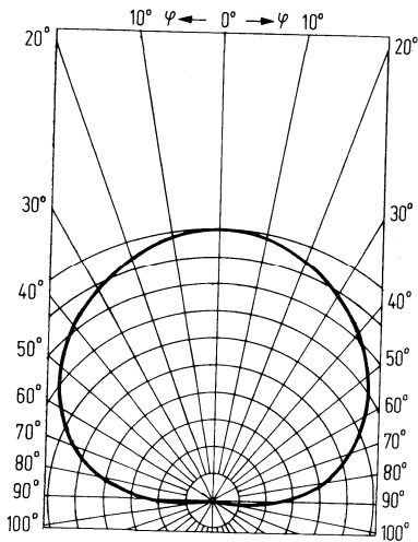
Richtcharakteristik I_P = f(\lambda)
