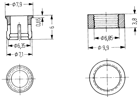
Befestigungs-Ring
