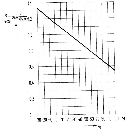
Strahlstärke \frac{I_n}{I_{e 25^\circ}} = f(T_U)
