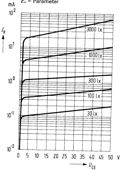
Fotostrom I_P = f(U_{CE}) E_V = \text{Parameter}
