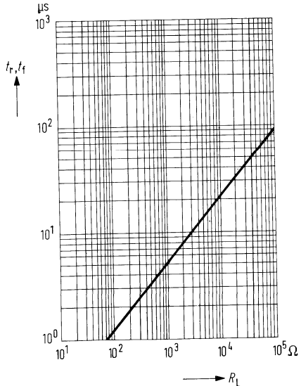
Anstiegszeit t_r = f(R_L) Abfallzeit t_f = f(R_L)
