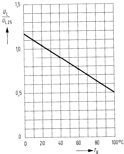
Temperaturabhängigkeit von U_L \frac{U_L}{U_{L, 25^\circ}} = f(T_U)
