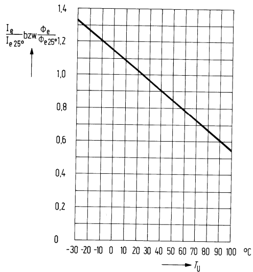
Strahlstärke \frac{I_e}{I_{e, 25^\circ}} bzw. \frac{\Phi_e}{\Phi_{e, 25^\circ, 1,2}} = f(T_U)
