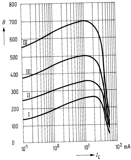
Stromverstärkung B = f(I_c) U_{CE} = 5 \text{ V}
