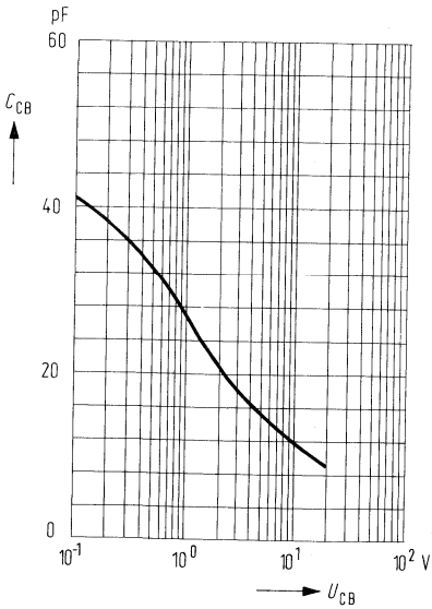
Kollektor-Basis-Kapazität C_{CB} = f(U_{CB})
