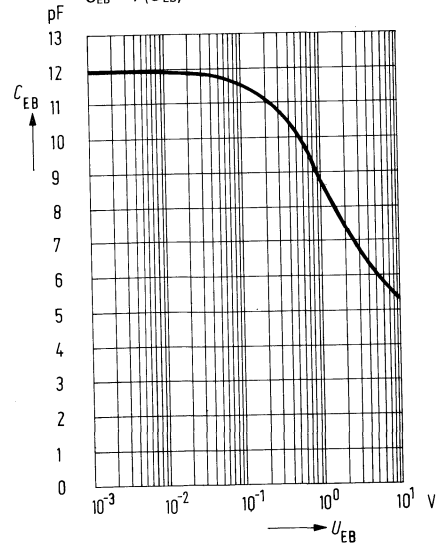
Emitter-Basis-Kapazität C_{EB} = f(U_{EB})
