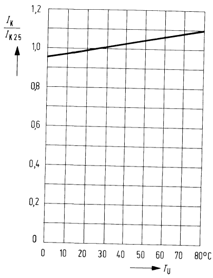
Kurzschlußstrom \frac{I_K}{I_{K 25^\circ}} = f(T_U)
