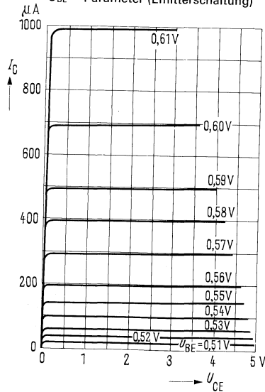
Ausgangskennlinie I_C = f(U_{CE}) U_{BE} = \text{Parameter (Emitterschaltung)}
