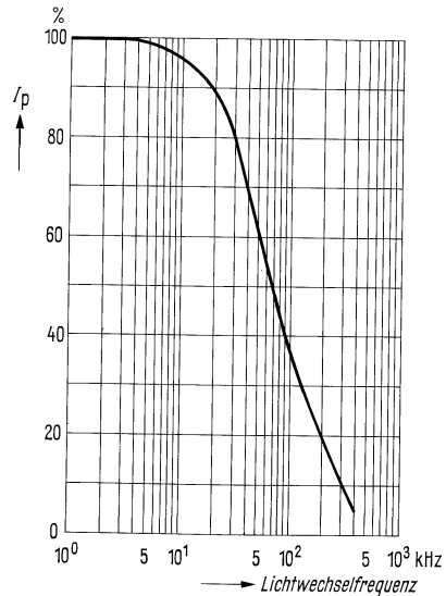
Mittlerer Fotostrom als Funktion der Lichtwechselfrequenz R_L = 1 \text{ k}\Omega ; E_v = 1000 \text{ lx}
