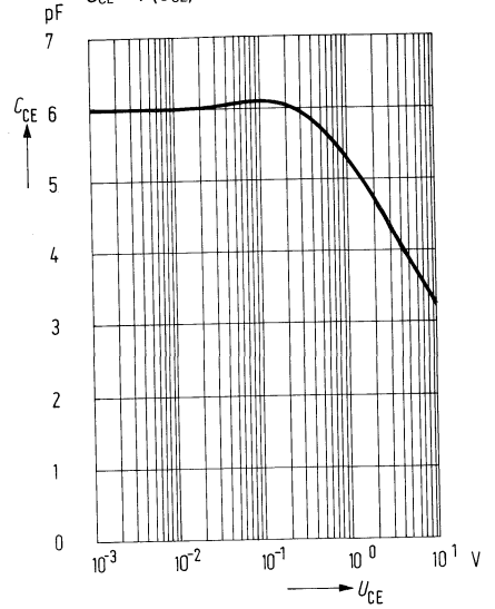
Kollektor-Emitter-Kapazität C_{CE} = f(U_{CE})
