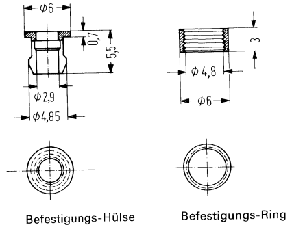
Befestigungs-Hülse
