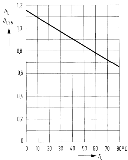
Leerlaufspannung \frac{U_L}{U_{L 25^\circ}} = f(T_U)
