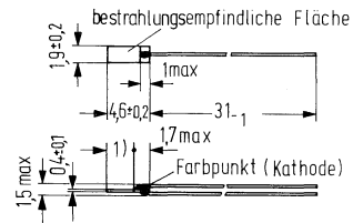
1) Auflagefläche 2,7min Gewicht etwa 0,2 g
