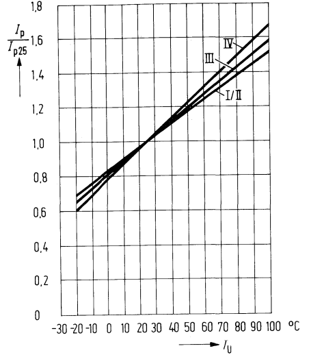
Fotostrom \frac{I_P}{I_{P 25^\circ}} = f(T_U)
