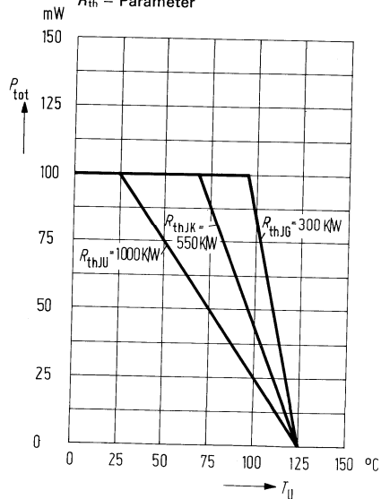
Verlustleistung P_{tot} = f(T_U) R_{th} = \text{Parameter}
