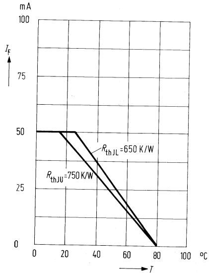
Maximal zul. Durchlaßstrom
