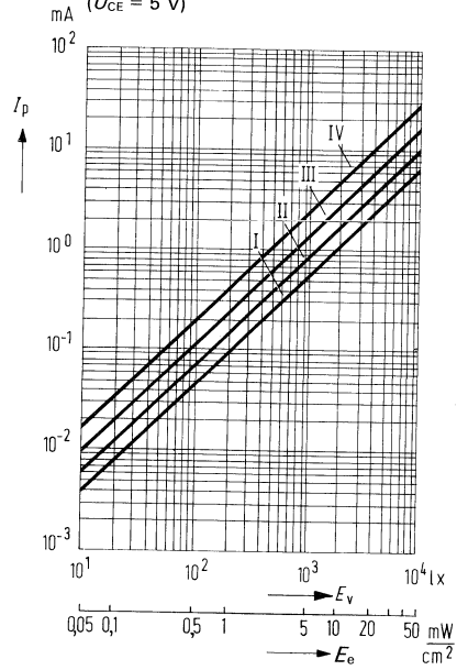
Fotostrom I_P = f(E_v) ( U_{CE} = 5 V )
