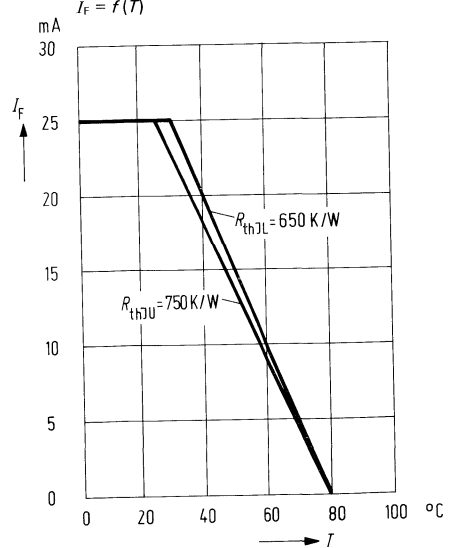
Maximal zulässiger Durchlaßstrom I_F = f(T)
