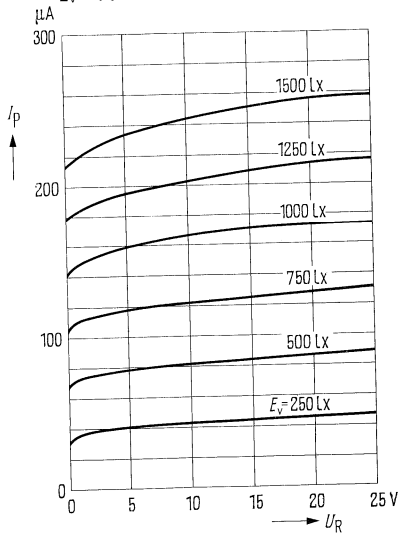
Kennlinienfeld I_P = f(U_R) E_v = \text{Parameter}
