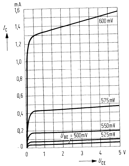
Ausgangskennlinien I_C = f(U_{CE}) U_{BE} = \text{Parameter}
