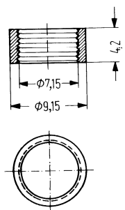
Befestigungs-Ring
