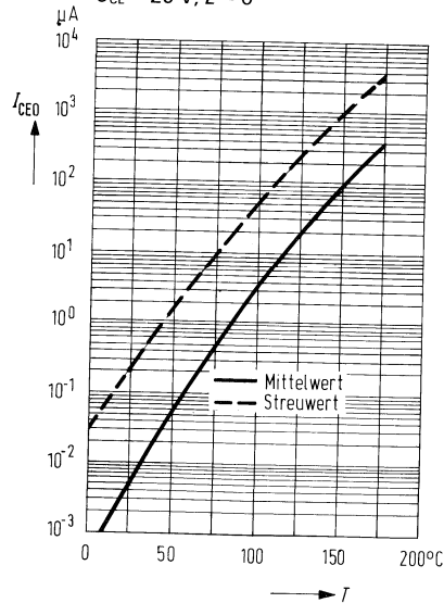
Dunkelstrom I_{CEO} = f(T) U_{CE} = 25 \text{ V}; E = 0
