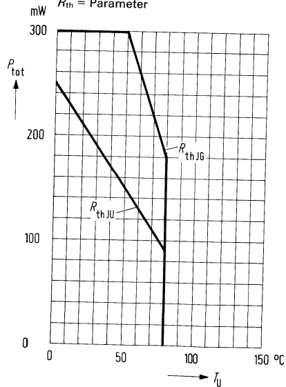
Verlustleistung P_{tot} = f(T_U) R_{th} = Parameter
