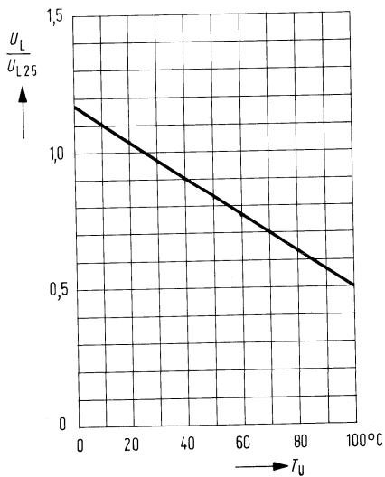
Temperaturabhängigkeit von U_L
