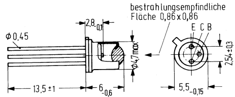
Gewicht etwa 1,5 g
