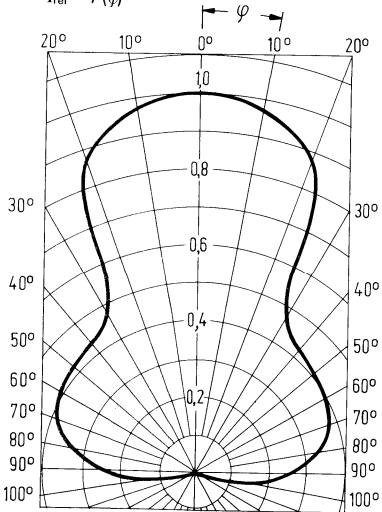
Abstrahlungscharakteristik
