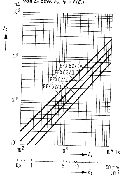
Fotostrom in Abhängigkeit von E_v bzw. E_e ; I_P = f(E_v)
