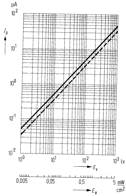
Fotostrom I_p = f(E_v)
