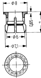
Befestigungs-Hülse
