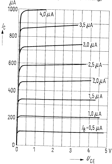
Ausgangskennlinie I_C = f(U_{CE}) I_B = \text{Parameter (Emitterschaltung)}
