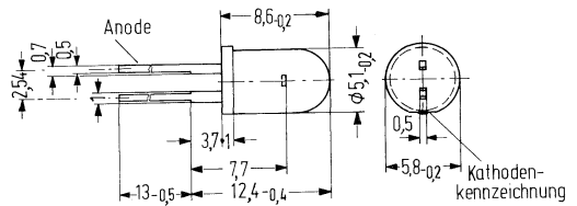
Gewicht etwa 0,2 g
