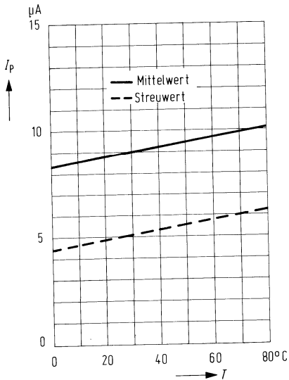
Fotostrom I_P = f(T) E_v = 1000\text{ lx} ; U_R = 1\text{ V}
