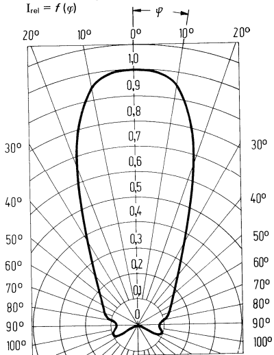
Abstrahlungscharakteristik
